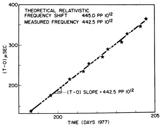
Fig. 20 - Cesium frequency via (T-O) slope
