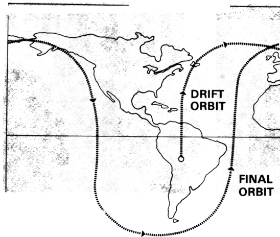
Fig. 5 - NTS-2 drift orbit
